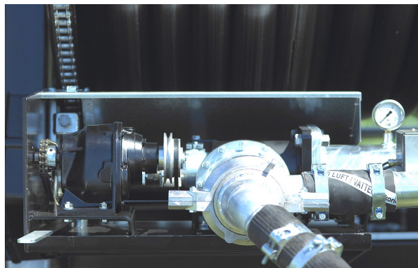
Turbindrivpaket med svirvlande anslutning
